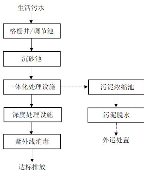
图 1 德庆肇水环保有限责任公司武垄镇污水厂工艺流程图
